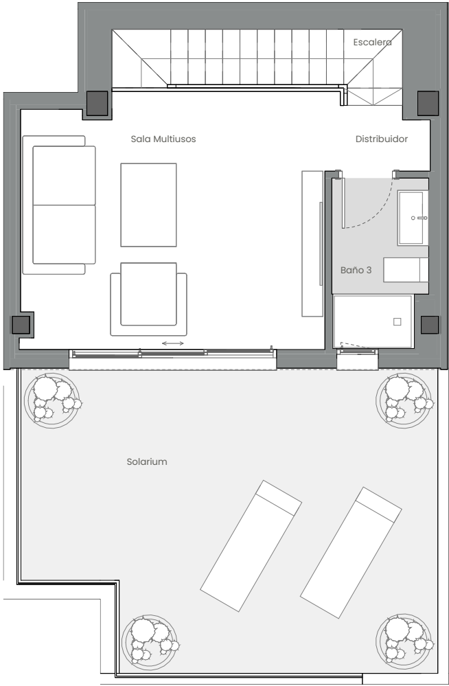
PLANTA SUPERIOR_P05
